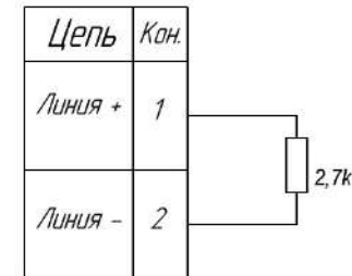
Рис.1. Схема подключения линии световых табло к согласующей коробке «КС-Т».
