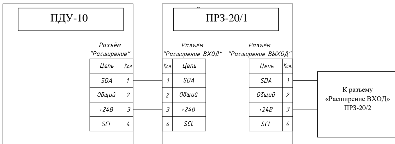
Рис. 1.2 Типовая схема подключения устройства
