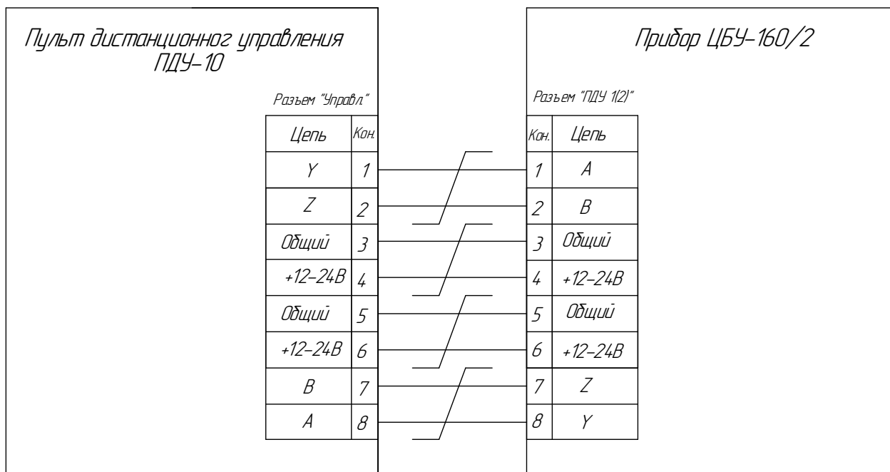
Рис. 1.6 Схема подключения пульта ПДУ-10 к ЦБУ-160/2
