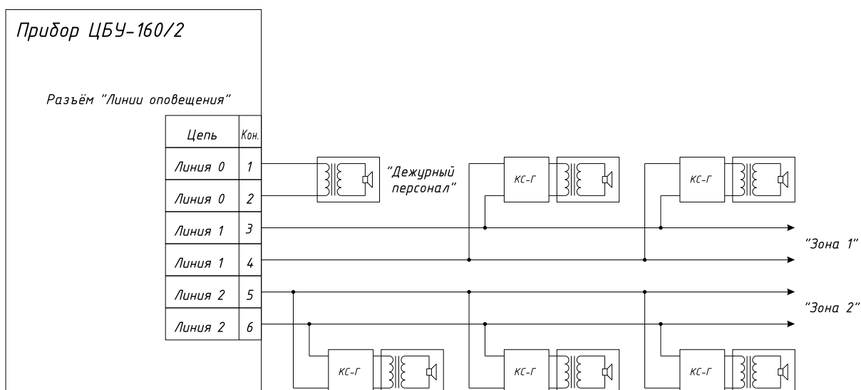
Рис. 1.3 Подключение громкоговорителей к линиям оповещения при суммарной нагрузке линии 100 Вт и более
