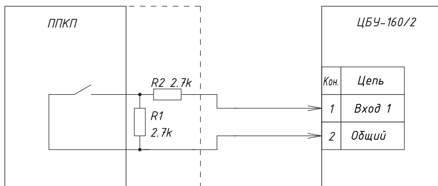
Рис. 1.4 Схема подключения ППКП (АУПС) к устройству ЦБУ-160/2.
