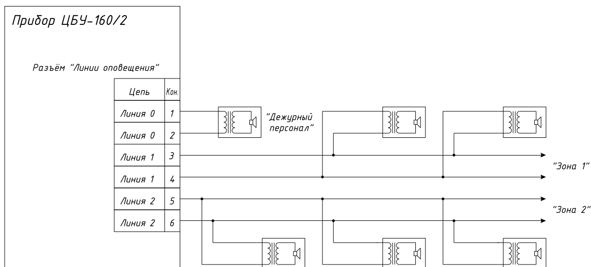
Рис. 1.2 Подключение громкоговорителей к линиям оповещения при суммарной нагрузке линии менее 100 Вт
