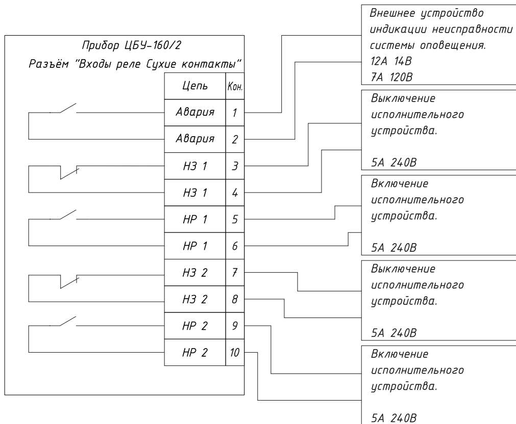
Рис. 1.10 Выходы реле "Сухие контакты"
