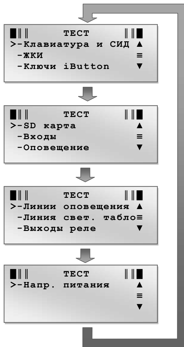
Рис. 2.35 Вид подменю ТЕСТ СИСТЕМЫ
