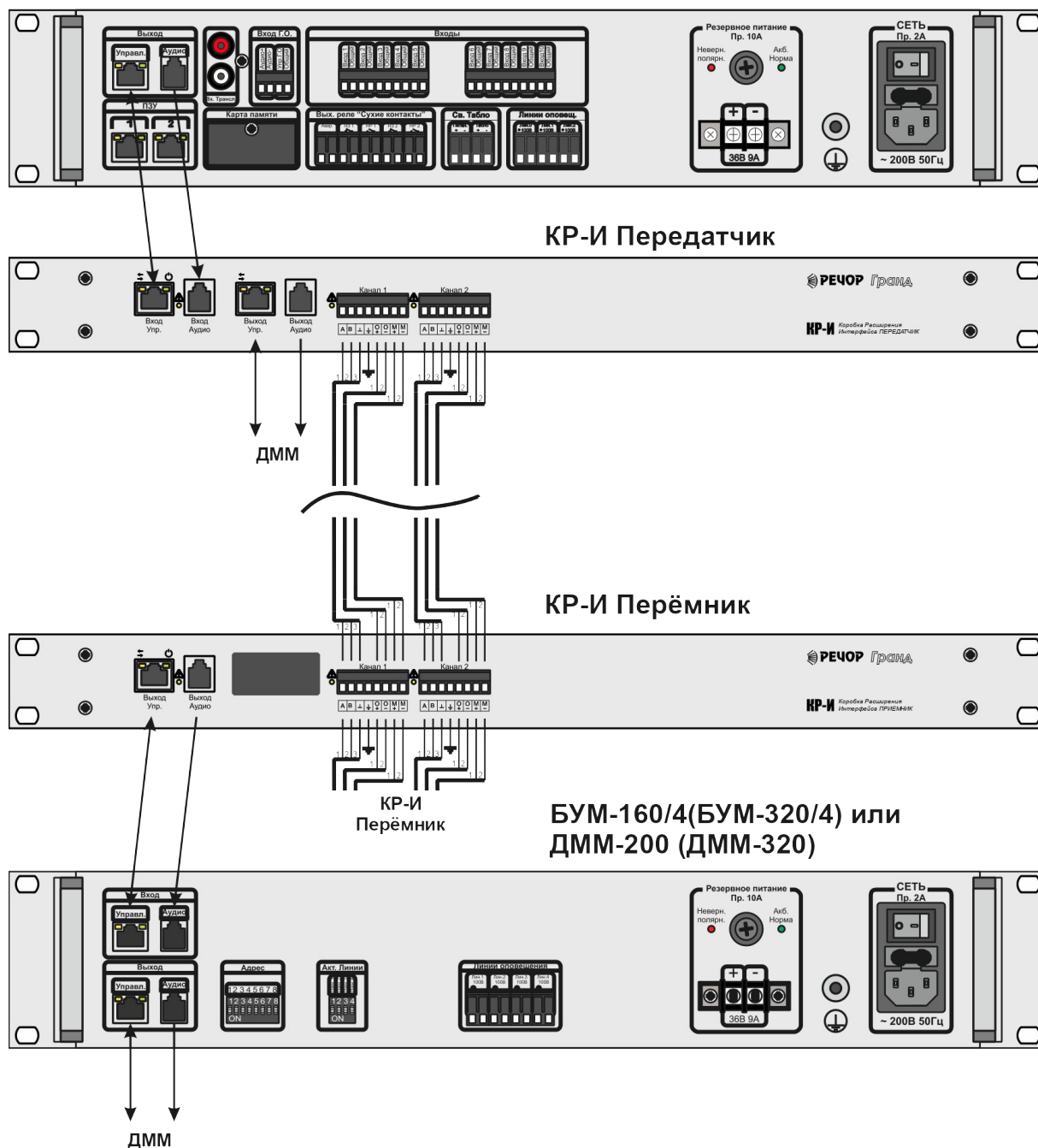
Рис. 1.13 Схема подключения КР-И
