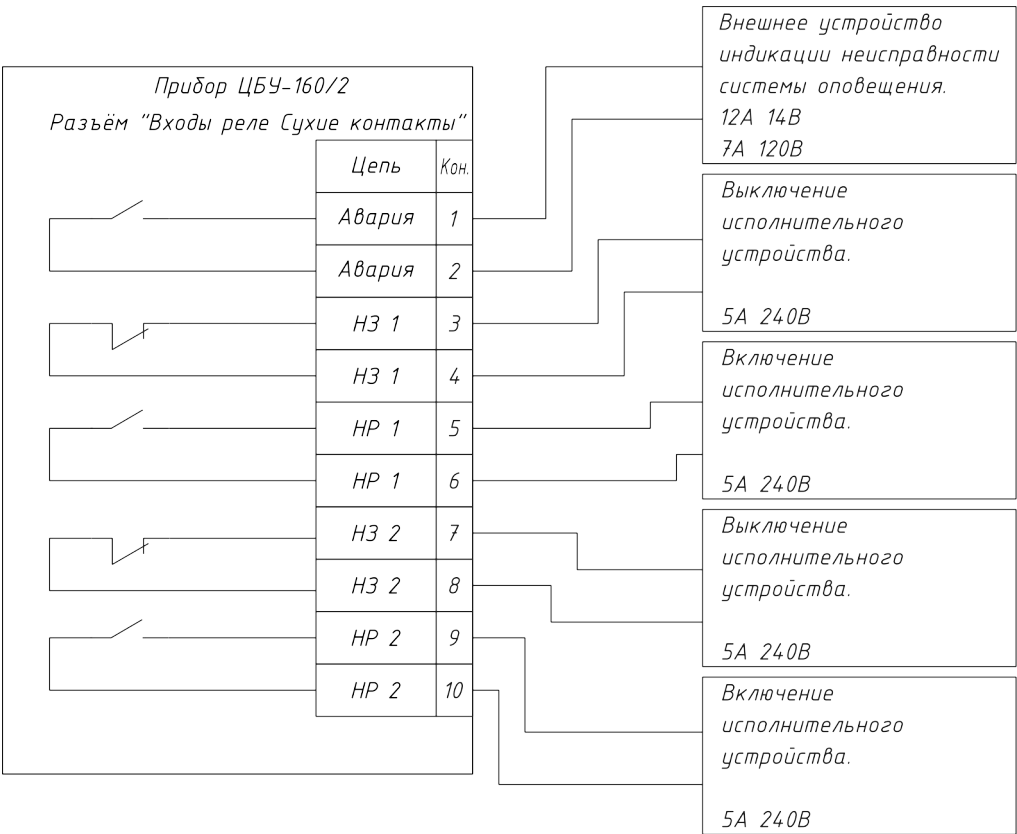
Рис. 1.9 Выходы реле "Сухие контакты". Разводка разъема
