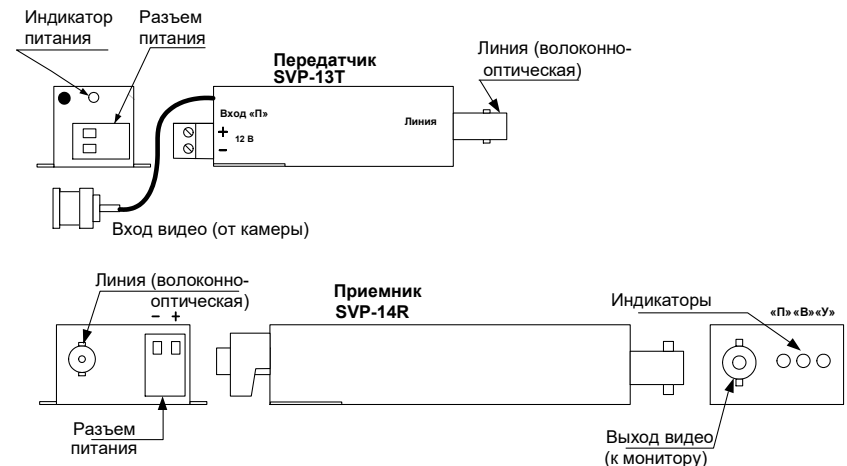
Рис. 1. Расположение разъемов и элементов индикации.
