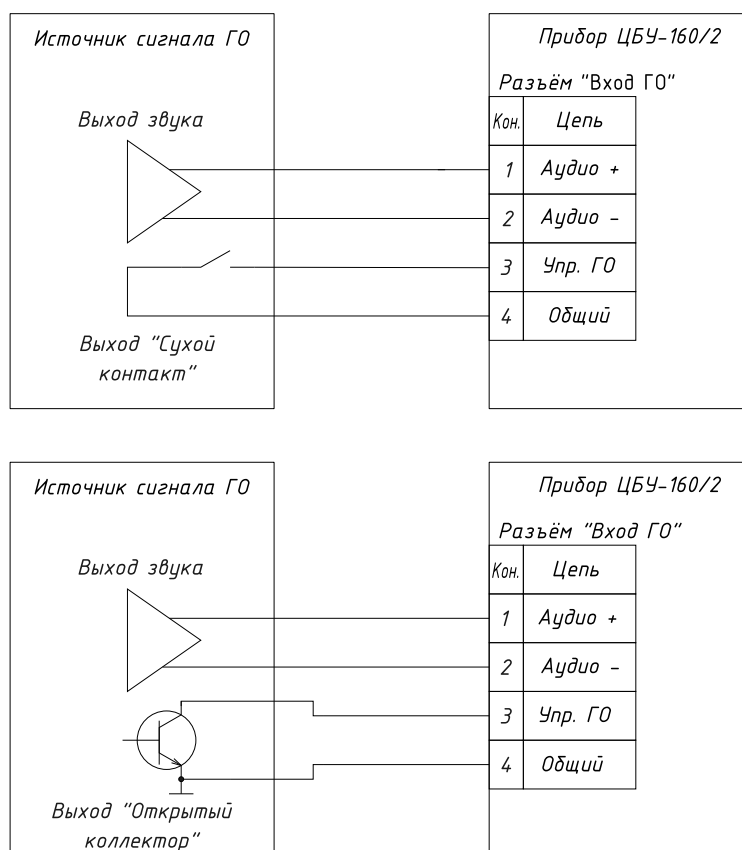
Рис. 1.7 Схемы подключения к источнику сообщения ГО МЧС
