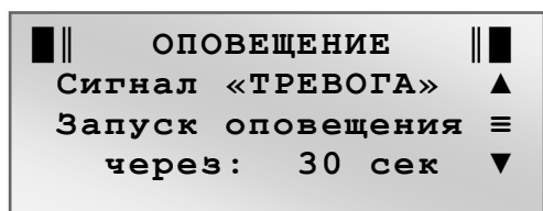
Рис. 2.10 Отображение при отработке интервала задержки запуска
