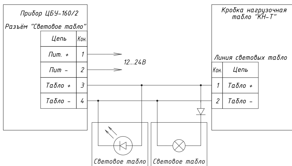
Рис. 1.9 Схема подключения световых табло
