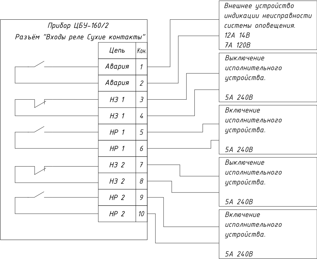
Рис. 1.10 Выходы реле "Сухие контакты"
