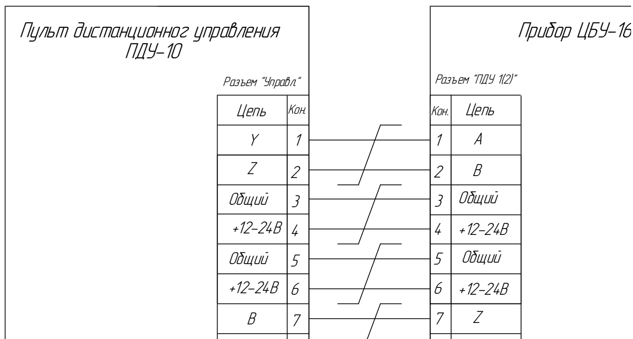
Рис. 1.6 Схема подключения пульта ПДУ-10 к ЦБУ-160/2
