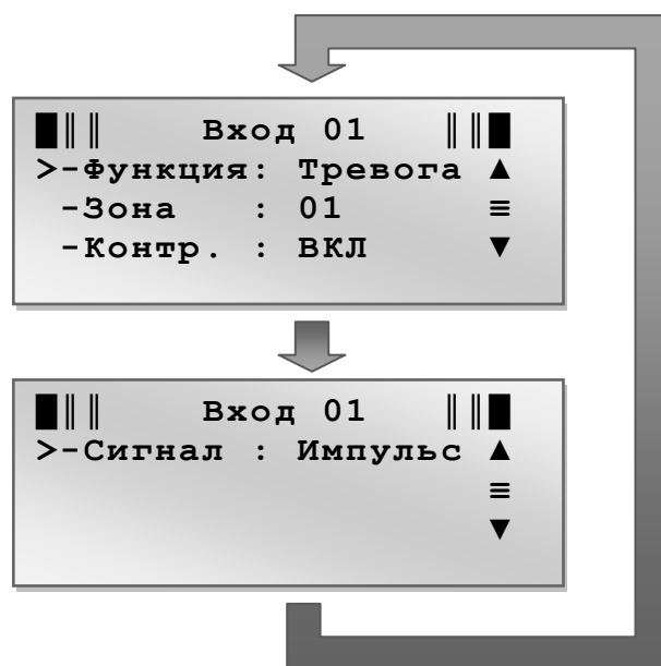
Рис. 2.18 Подменю Настройка Входа
