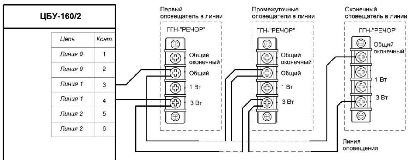
Рис. 1.2 Подключение громкоговорителей марки «РЕЧОР» к линиям оповещения.
