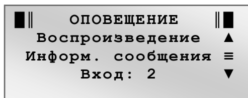
Рис. 2.13 Вид окна режима работы ОПОВЕЩЕНИЕ при воспроизведении информационного сообщения
