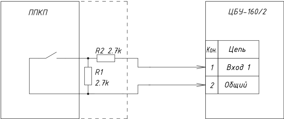
Рис. 1.5 Схема подключения ППКП (АУПС) с контролем целостности шлейфа
