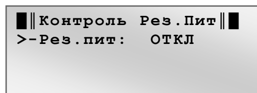
Рис. 2.33 Окно подменю "Рез. Пит."
