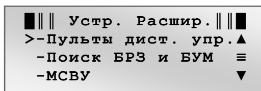
Рис. 2.21 Окно подменю УСТРОЙСТВА РАСШИРЕНИЯ
