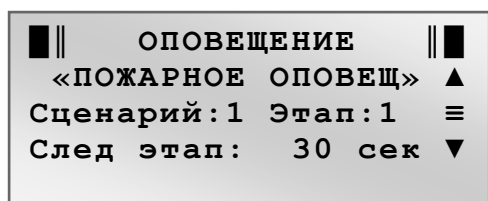
Рис. 2.11 Вид окна режима работы ОПОВЕЩЕНИЕ
