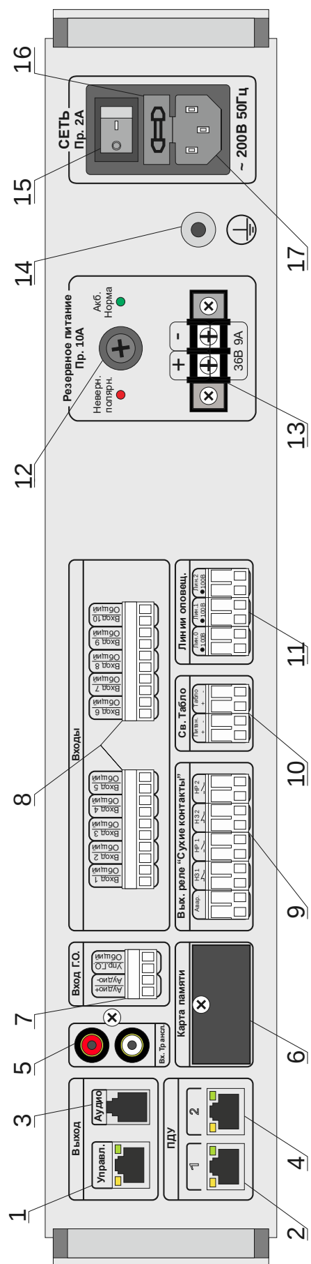
Рис. 2.40 Вид задней панели
