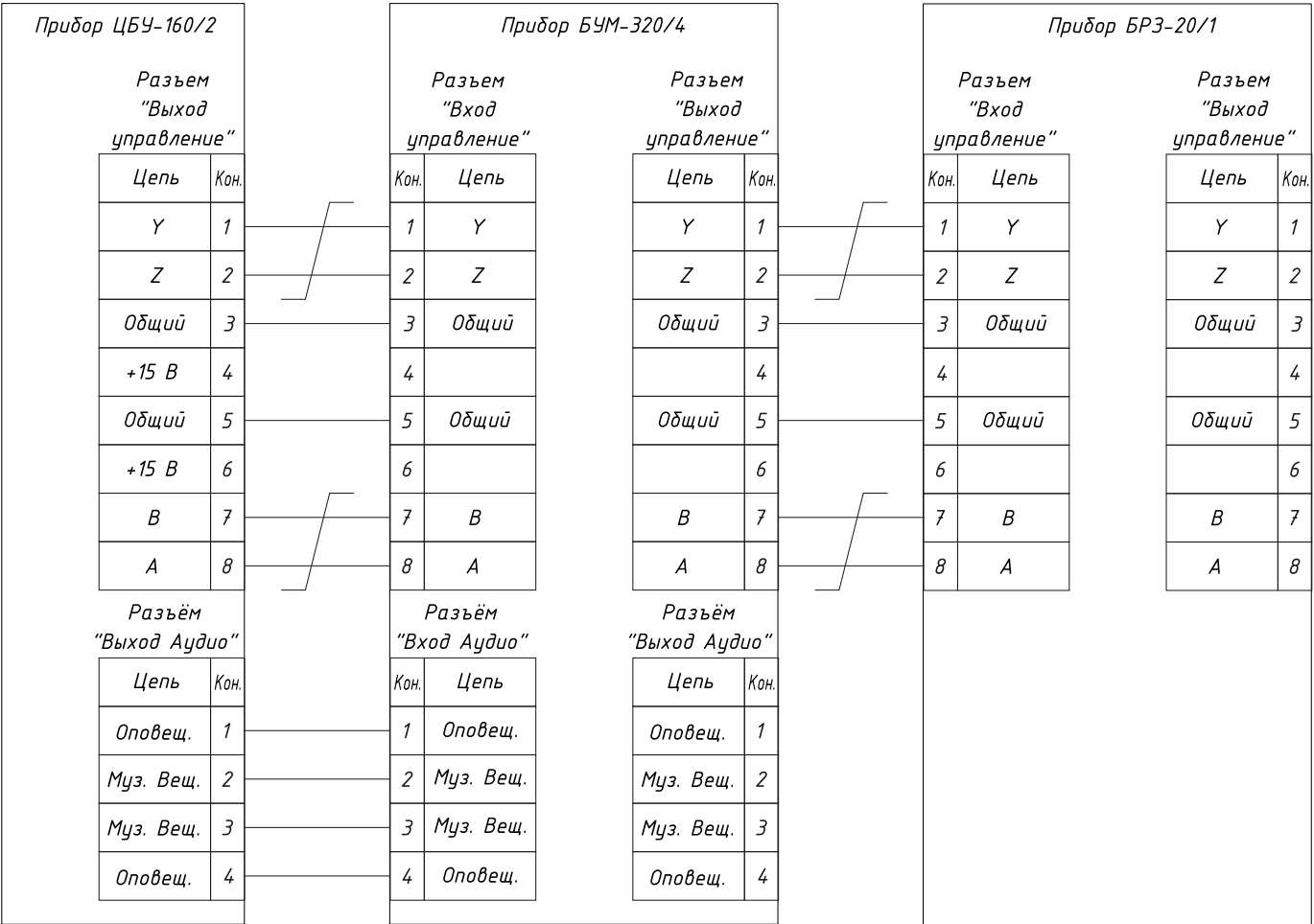
Рис. 1.11 Пример подключения к ЦБУ-160/2 дополнительных БУМ и БРЗ по шине расширения
