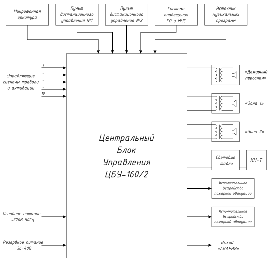
Рис. 1.1 Схема подключения ЦБУ-160/2 в автономном режиме работы
