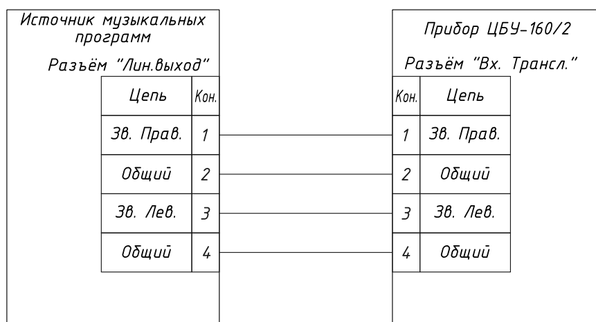
Рис. 1.8 Схема подключения к источнику музыкальных программ
