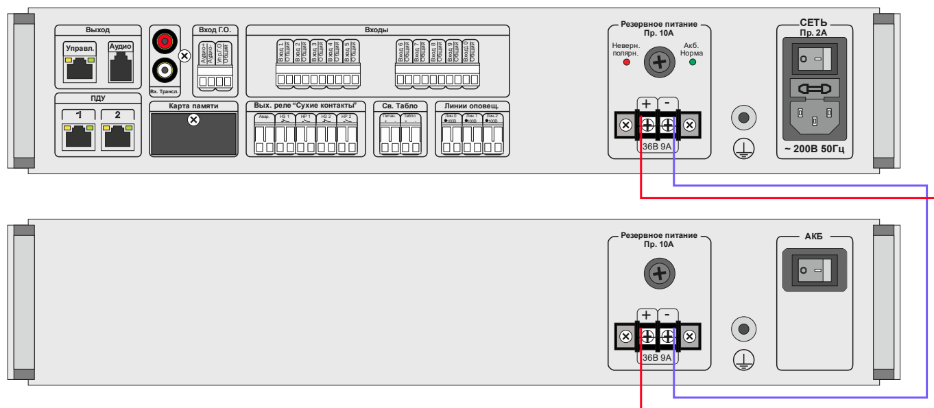
Рис. 2.38 Подключение к ЦБУ-160/2 блока резервного питания БРП-36/07
