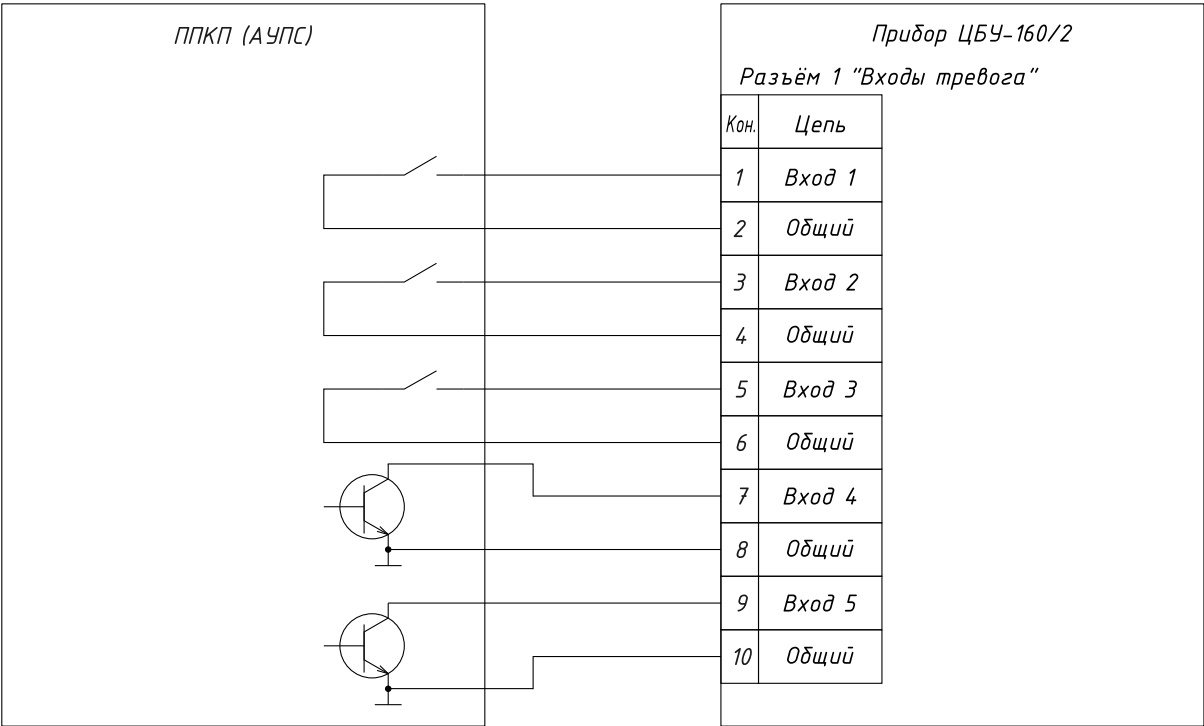
Рис. 1.4 Схема подключения ППКП (АУПС) к устройству ЦБУ-160/2.
