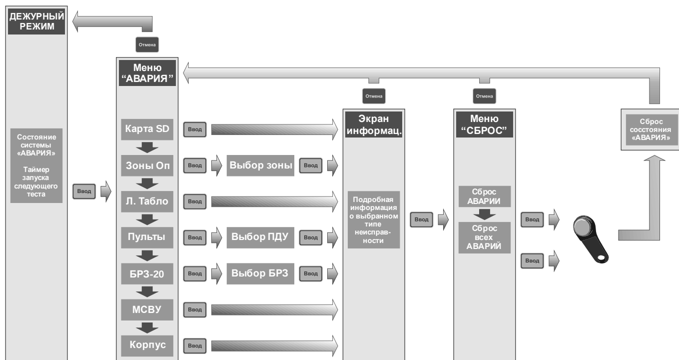
Рис. 2.4 Структура меню АВАРИЯ
