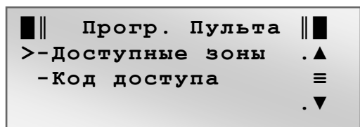
Рис. 2.24 Окно подменю ПРОГР. ПУЛЬТА
