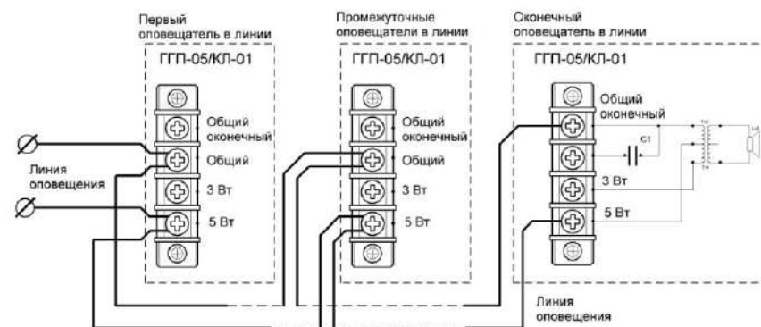
Рис.1. Схема подключения потолочных оповещателей «РЕЧОР» в линию.
