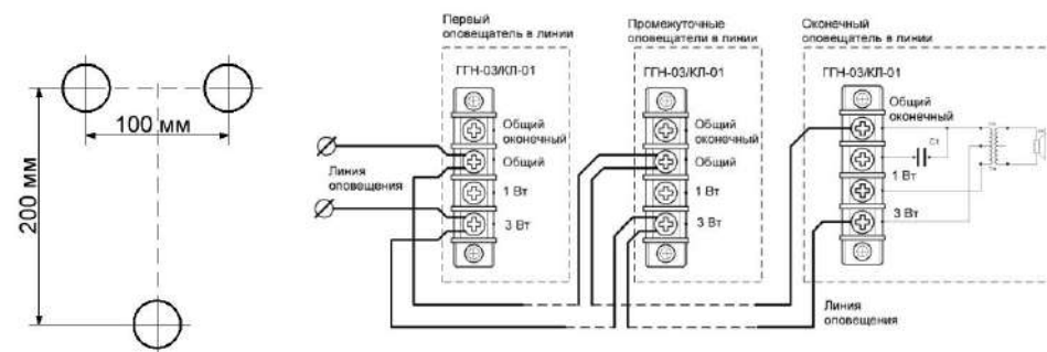
Рис.2. Схема подключения оповещателей «РЕЧОР» в линию.
